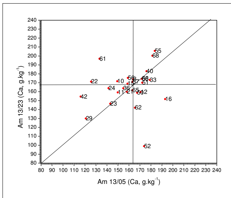
Figura 10. Diagrama de dispersão para a análise de cálcio (Ca) da amostra de misturar mineral repetida, 13/05 e 13/13.
